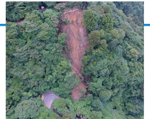
高さ60メートルにわたって崩落している斜面
